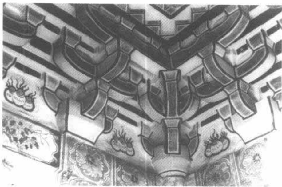
第96图 杭州开化寺六和塔室内斗拱
