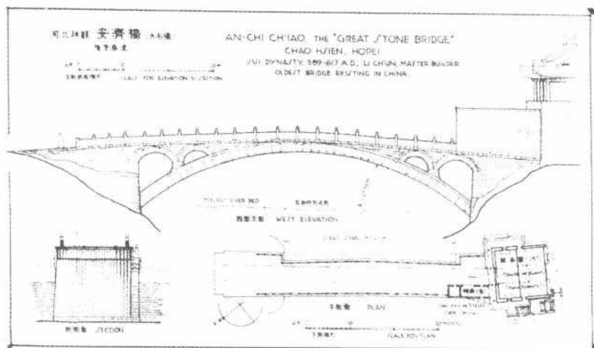
第 34 图 安济桥平、立、剖平面
