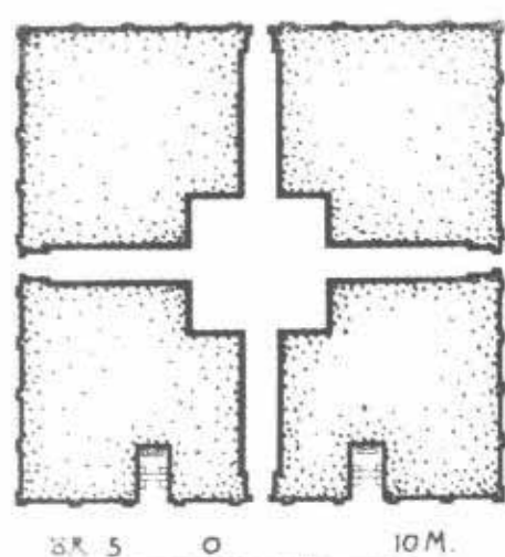
西安慈恩寺大雁塔平面圖
