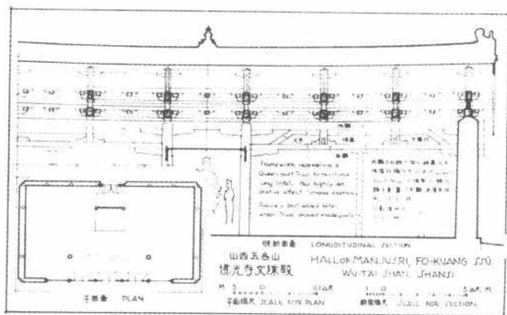
第 48 图 山西五台山佛光寺文殊殿梁架构造
