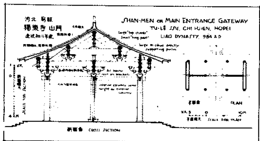
第 43 图 独乐寺山门平面及剖面
