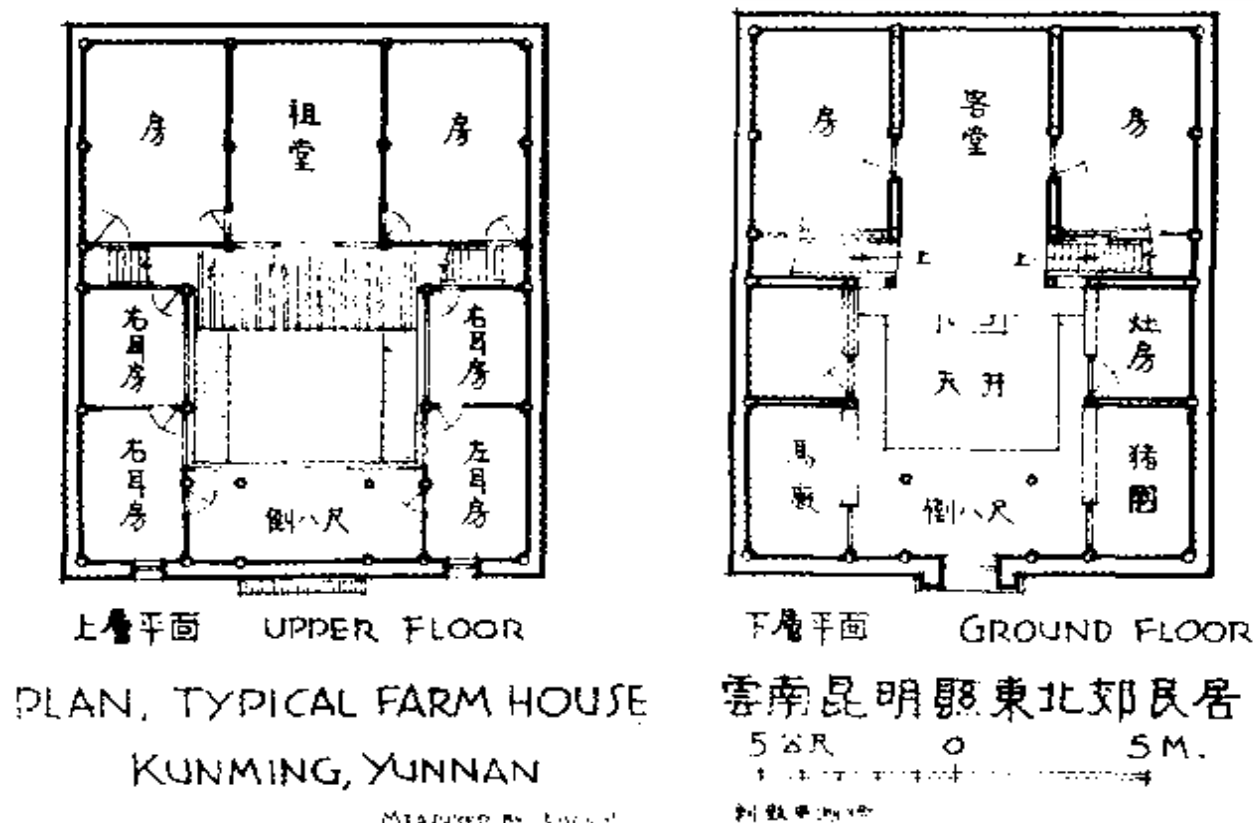
第 177 图 云南昆明县东北郊民居平面图
