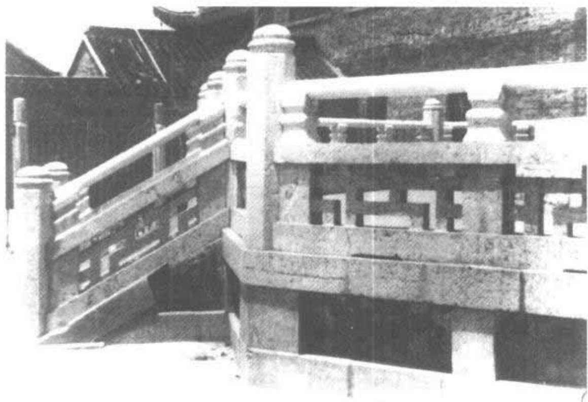
第80图 舍利塔石阶及勾栏
