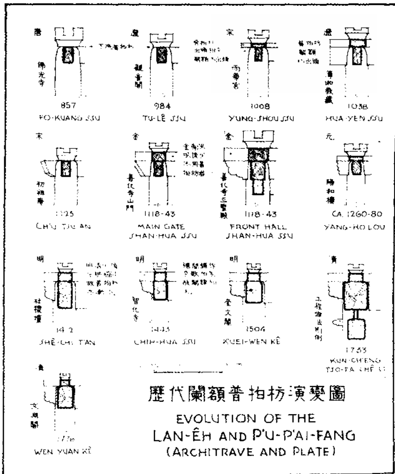
第 193 图 历代闌額、普拍枋演变图
