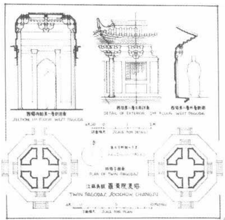
第 84 图 江苏吴县罗汉院双塔平面、断面、立面图
