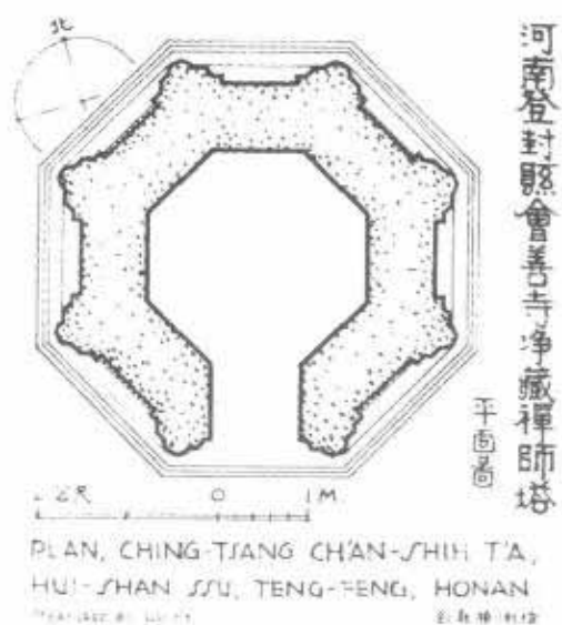
第31图 净藏禅师塔平面
