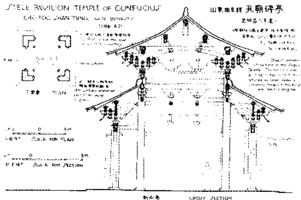
第78图 山东曲阜县孔庙碑断面及平面
