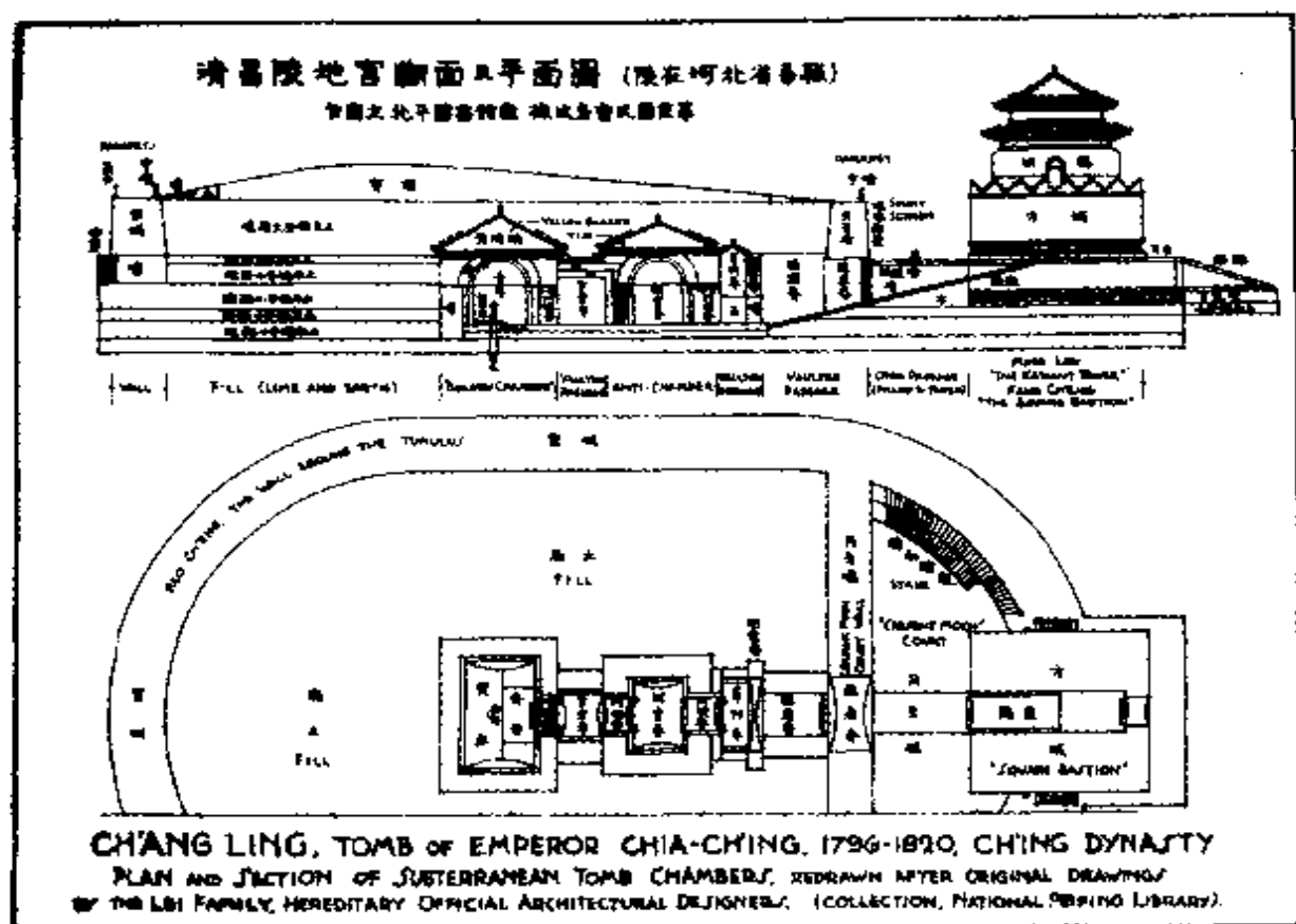
第 164 图 清昌陵地宫断面及平面图
