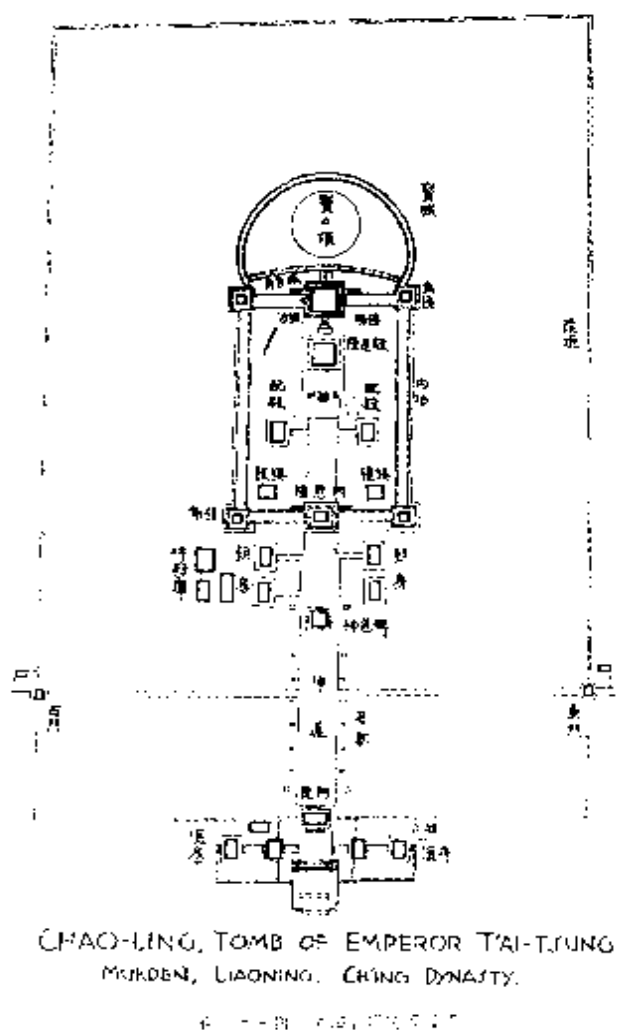
第 161 图 沈阳清昭陵平面图
