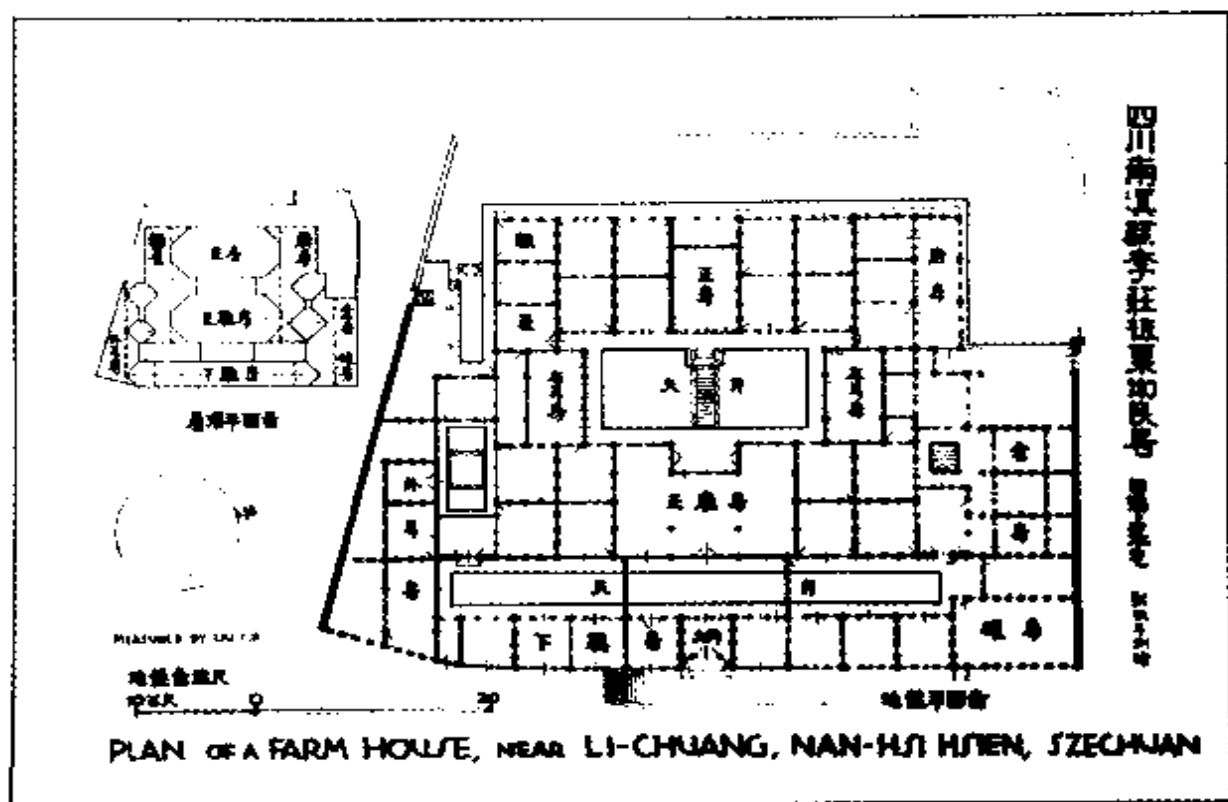
第174图 四川南溪李庄民居平面
