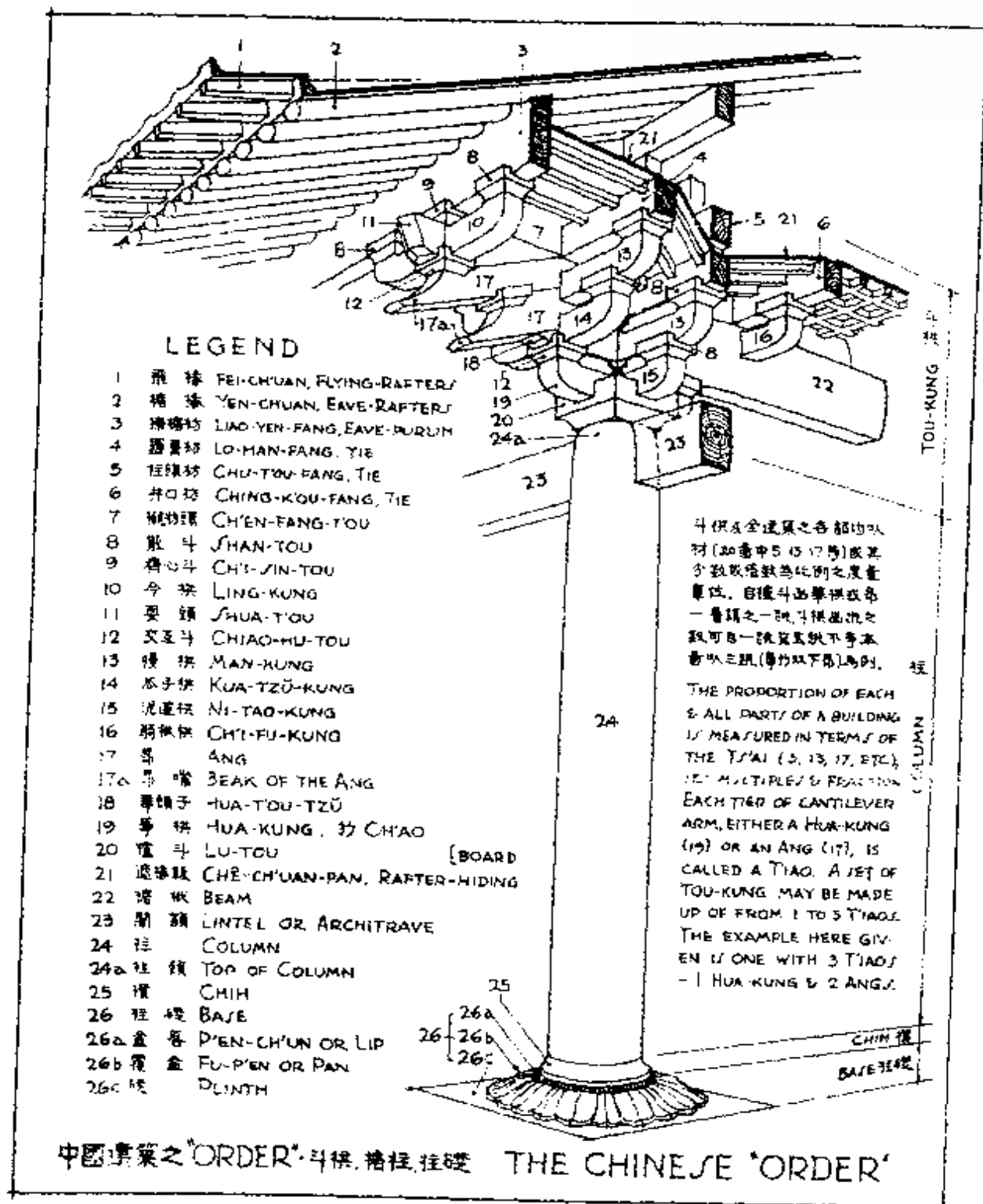
第 2 图 中国建筑之“ORDER”
