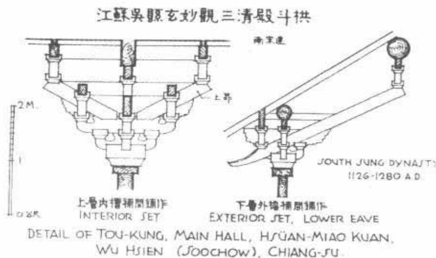
第77图 玄妙观三清殿斗拱
