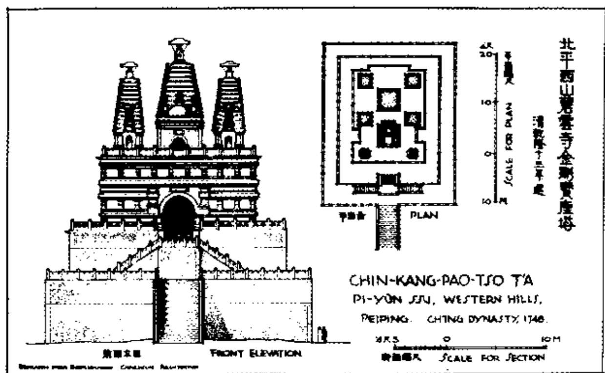
第 171 图 北京碧云寺金刚宝座塔
