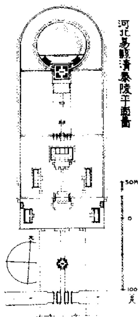
第 162 图 河北易县清泰陵平面图
