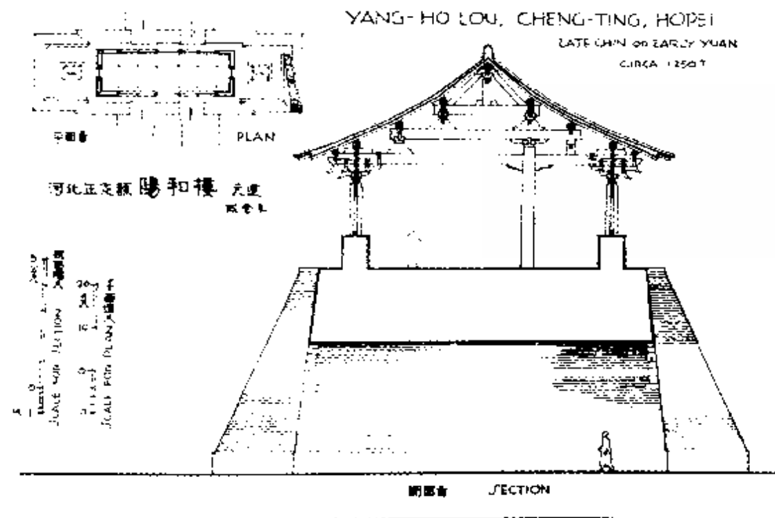
第 108 图 河北正定阳和楼剖面及平面
