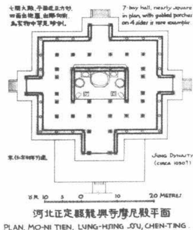
第 51 图 龙兴寺摩尼殿平面
