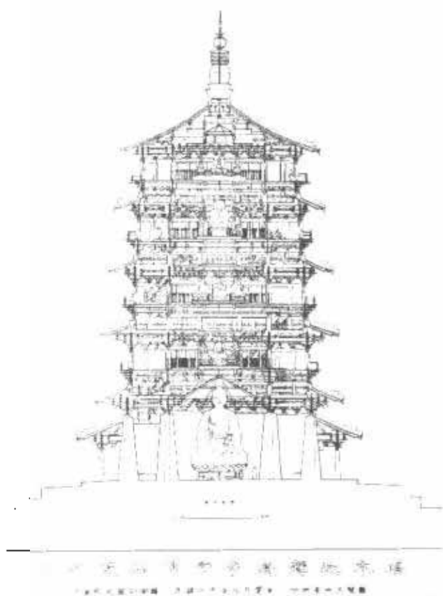
第 64 图 山西应县佛宫寺释迦塔断面图
