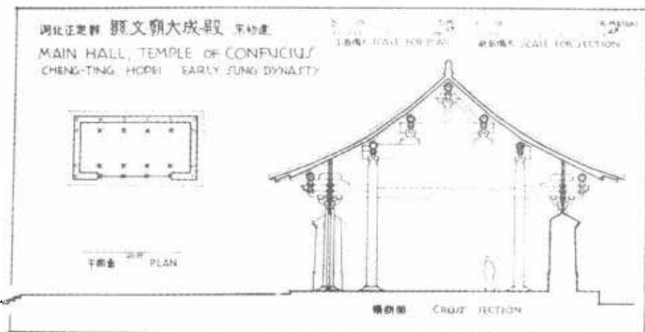
第 37 图 正定文庙大成殿平、剖面
