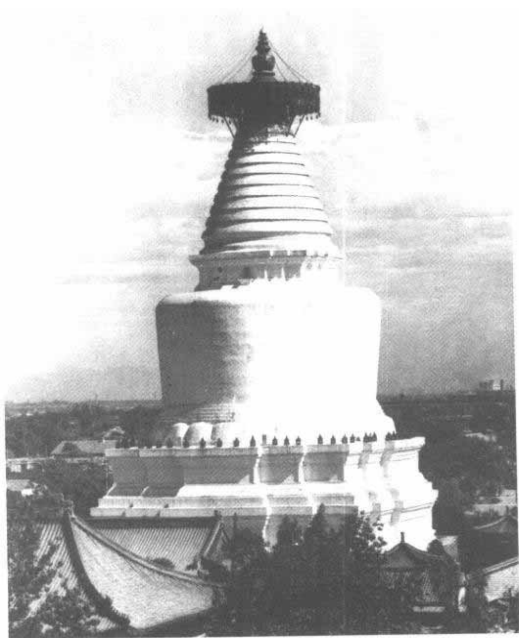
第 121 图 北京妙应寺白塔
