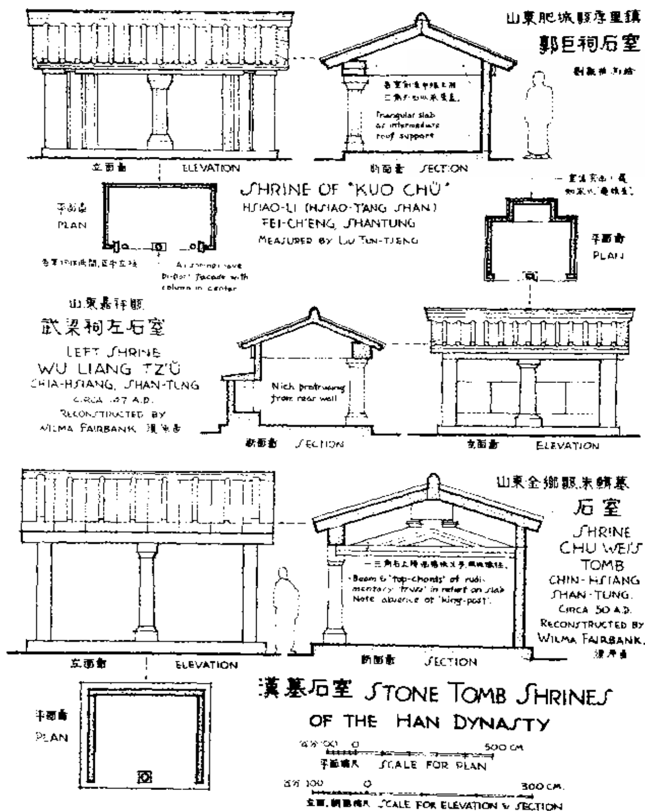
第 6 图 汉墓石室
