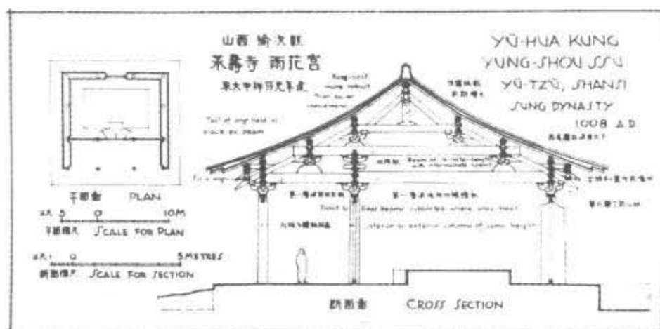
第 47 图 永寿寺雨花宫剖面及平面
