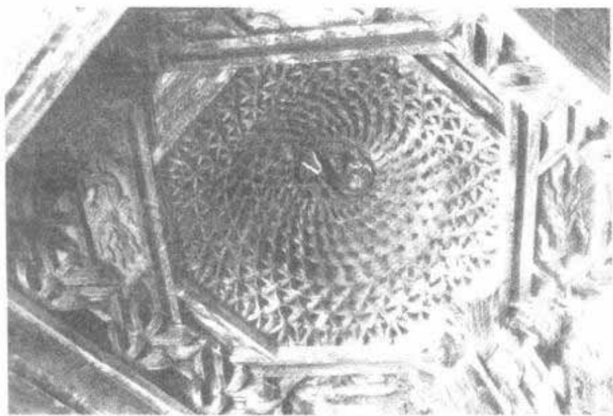
第 127 图 开福寺大雄宝殿藻井
