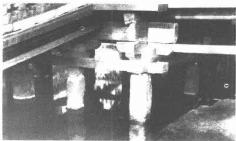
第 57 图 晋祠圣母庙飞梁
