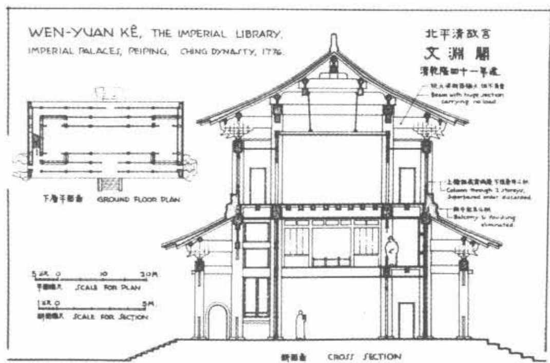
第 150 图 北京故宫文渊阁平面及剖面
