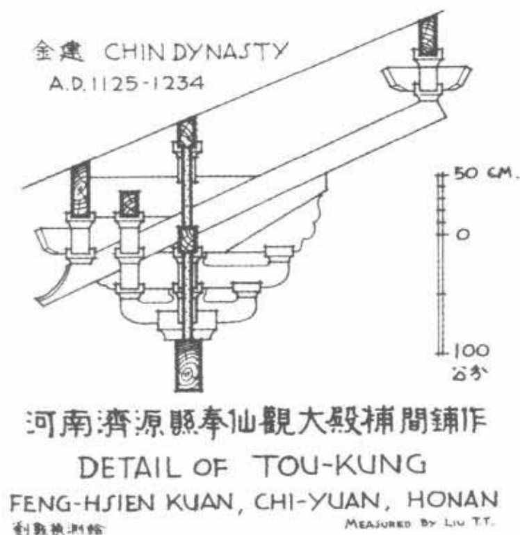
第 75 图 奉仙观大殿斗拱
