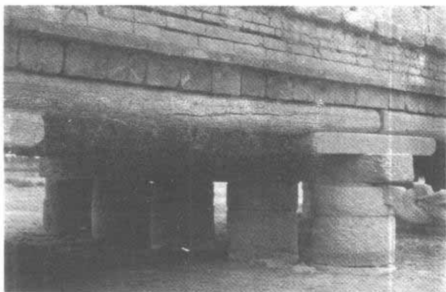
第 183 图 灞桥石轴石梁
