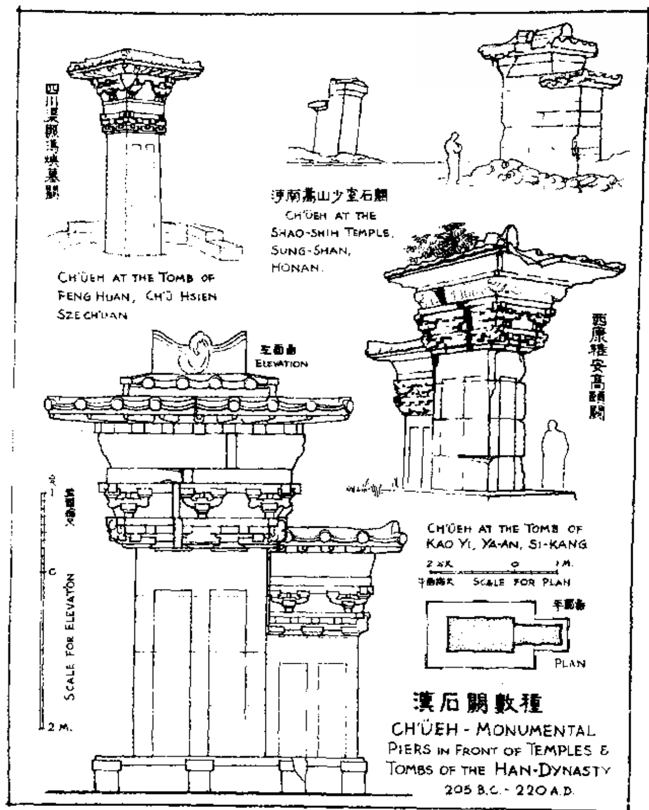
第7图 汉石阙数种
