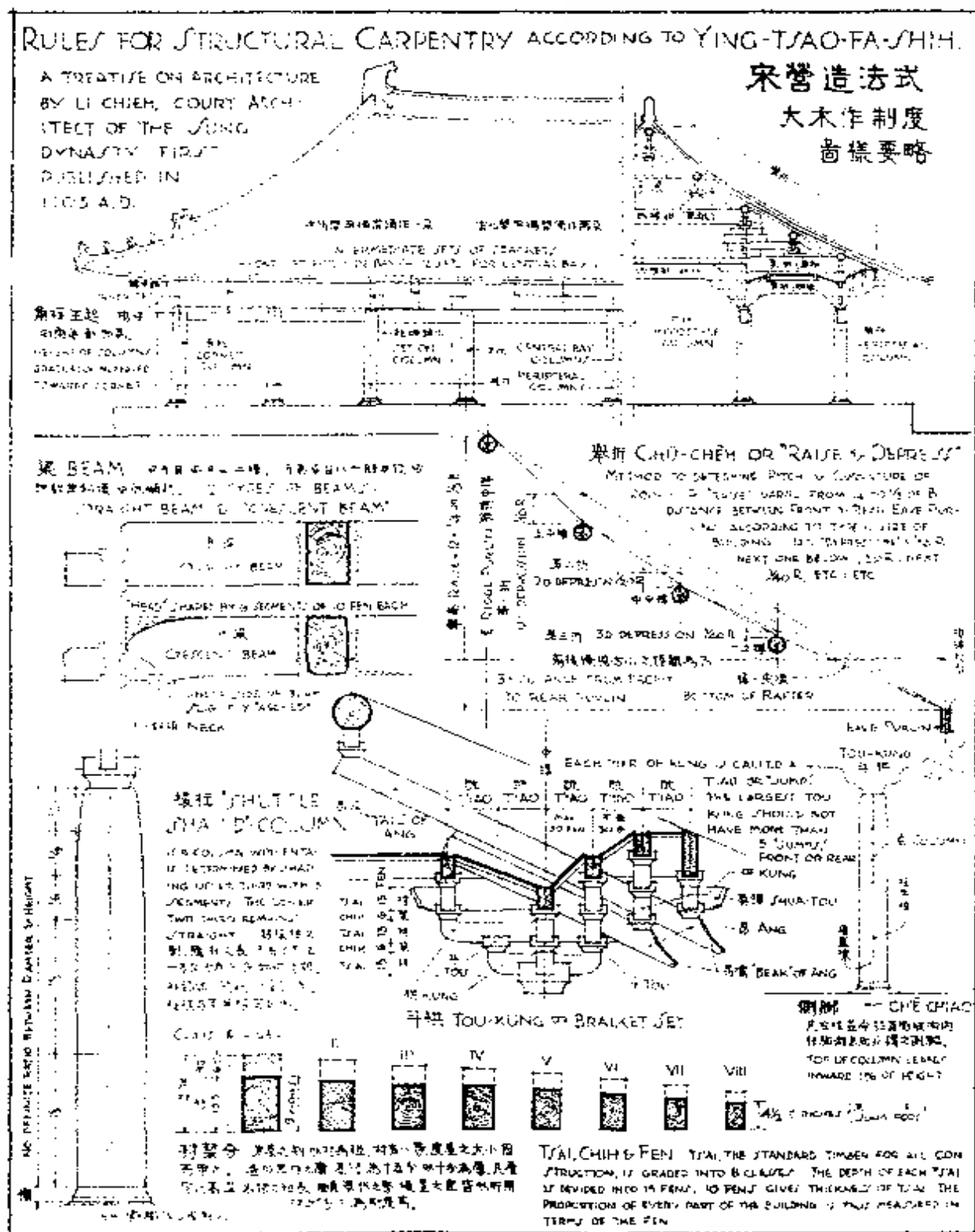
第3图 宋《营造法式》大木作制度图样要略
