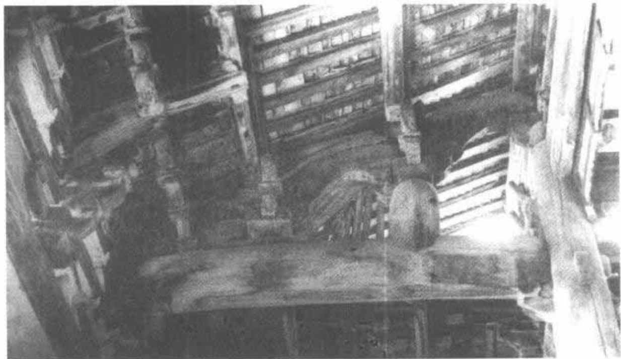
第 113 图 延福寺大殿斗拱
