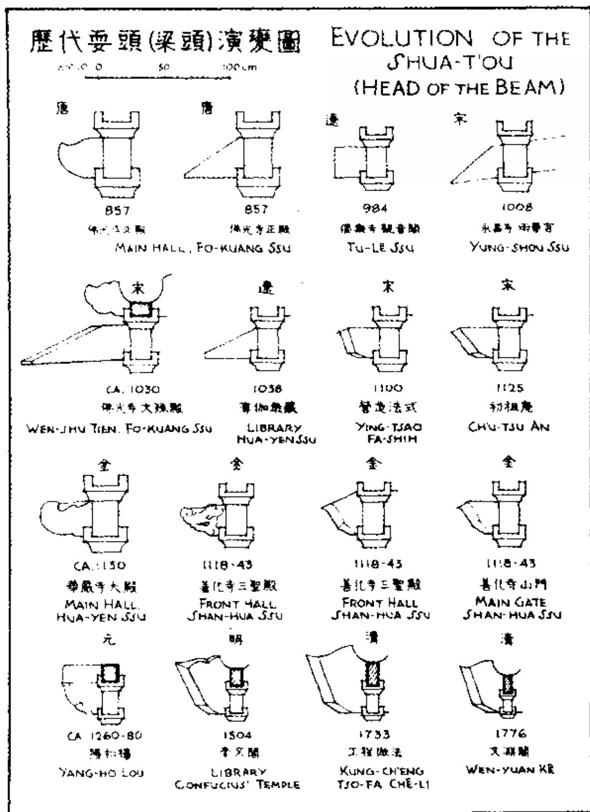
第 194 图 历代耍头演变图
