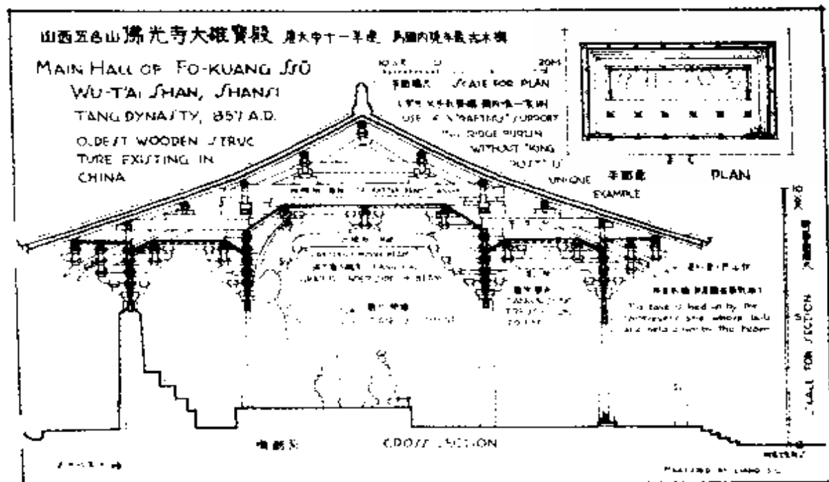
第20图 山西五台山佛光寺大雄宝殿断面及平面图
