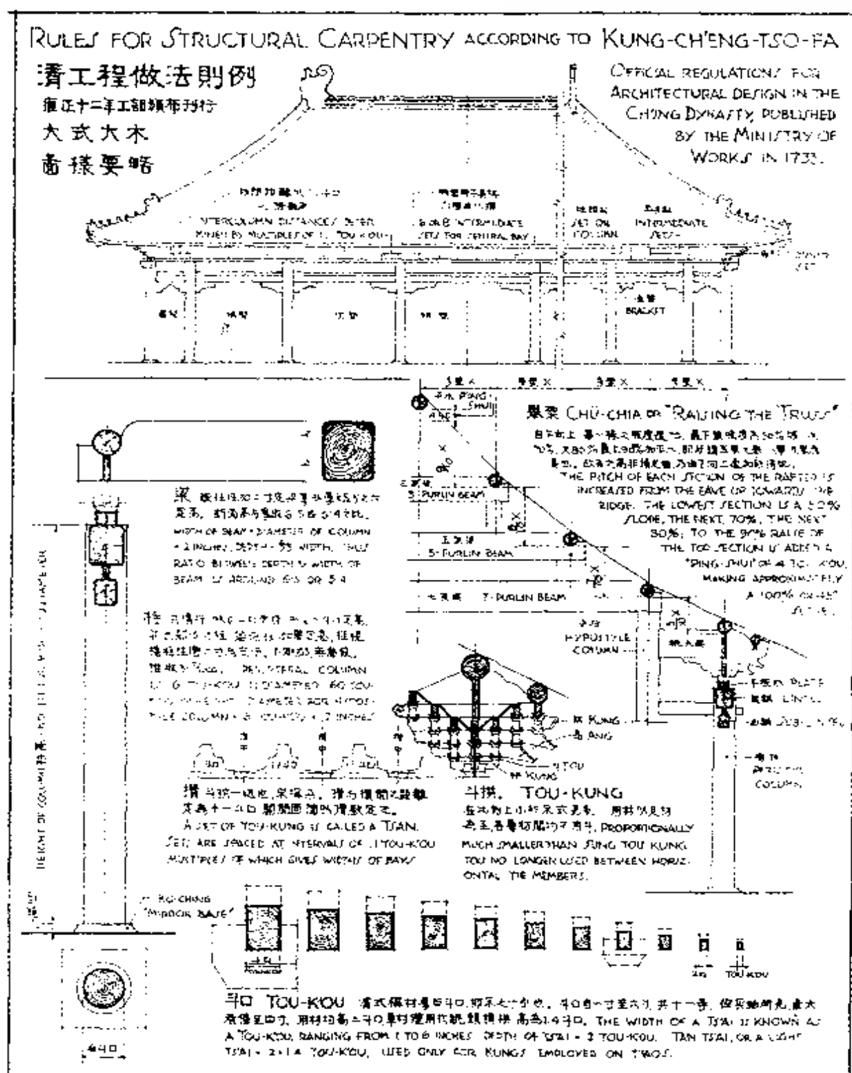
第 4 图 清工部《工程做法則例》大式木作图样要略
