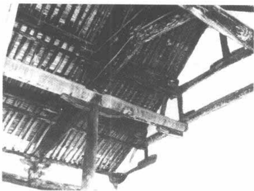
第 115 图 山西赵城县广胜寺下寺前殿梁架(元) (前后用三椽斜挑大梁交于平梁正中之下)
