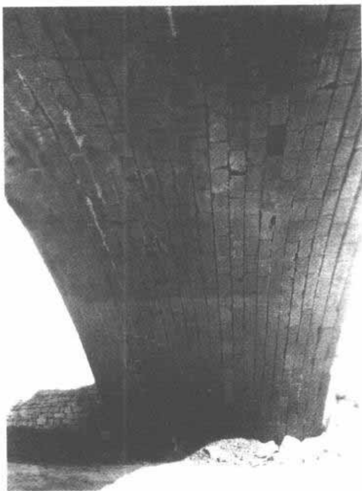
第 33 图 安济桥券底
