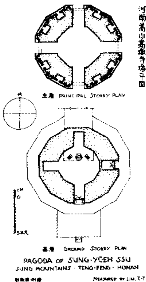
第 14 图 河南嵩山嵩岳寺塔平面
