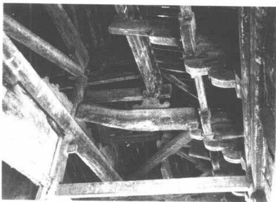
第 53 图 龙兴寺转轮藏梁架
