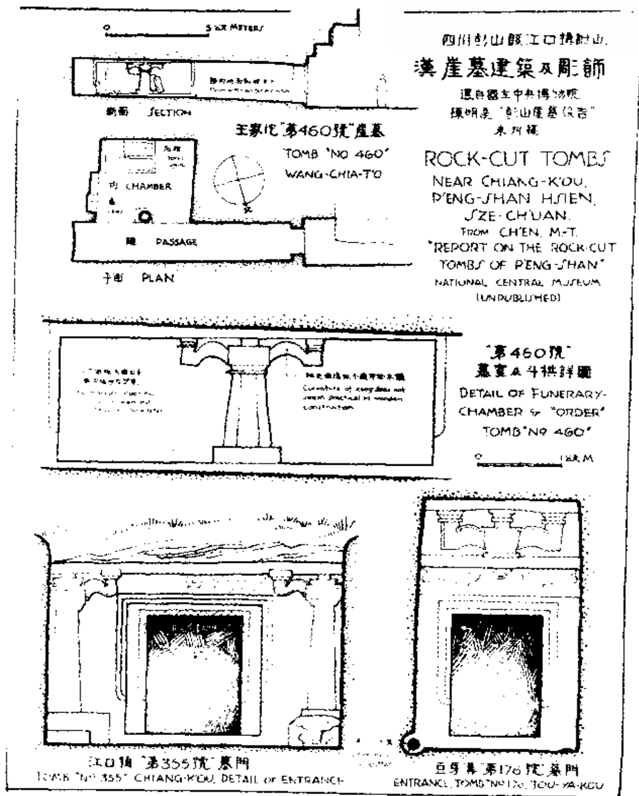
第 8 图 汉崖墓建筑及雕饰
