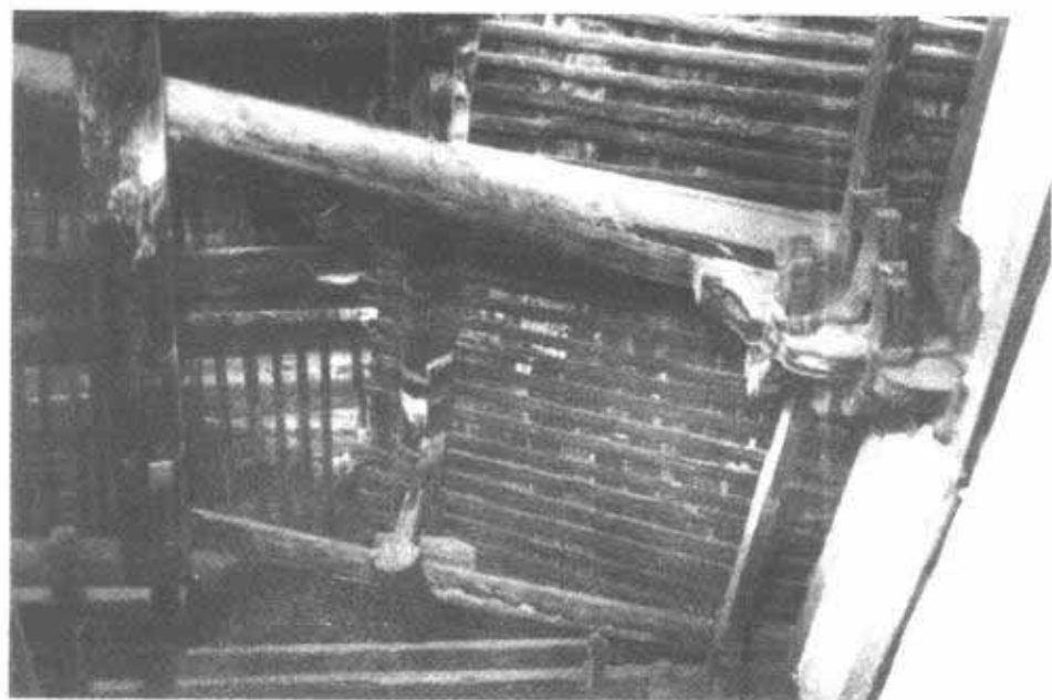
第 116 图 山西赵城县广胜寺上寺前殿梁架
