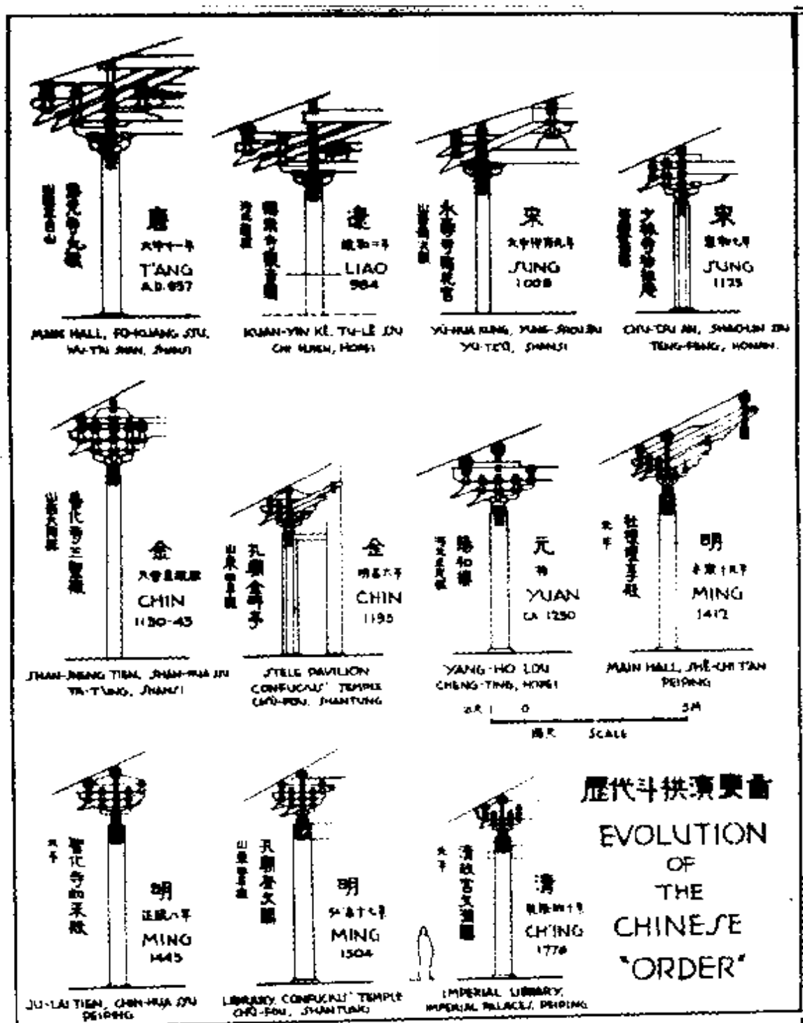
第 189 图 历代斗拱演变图
