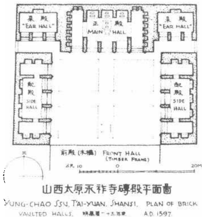
第 145 图 山西太原永祚寺砖殿平面
