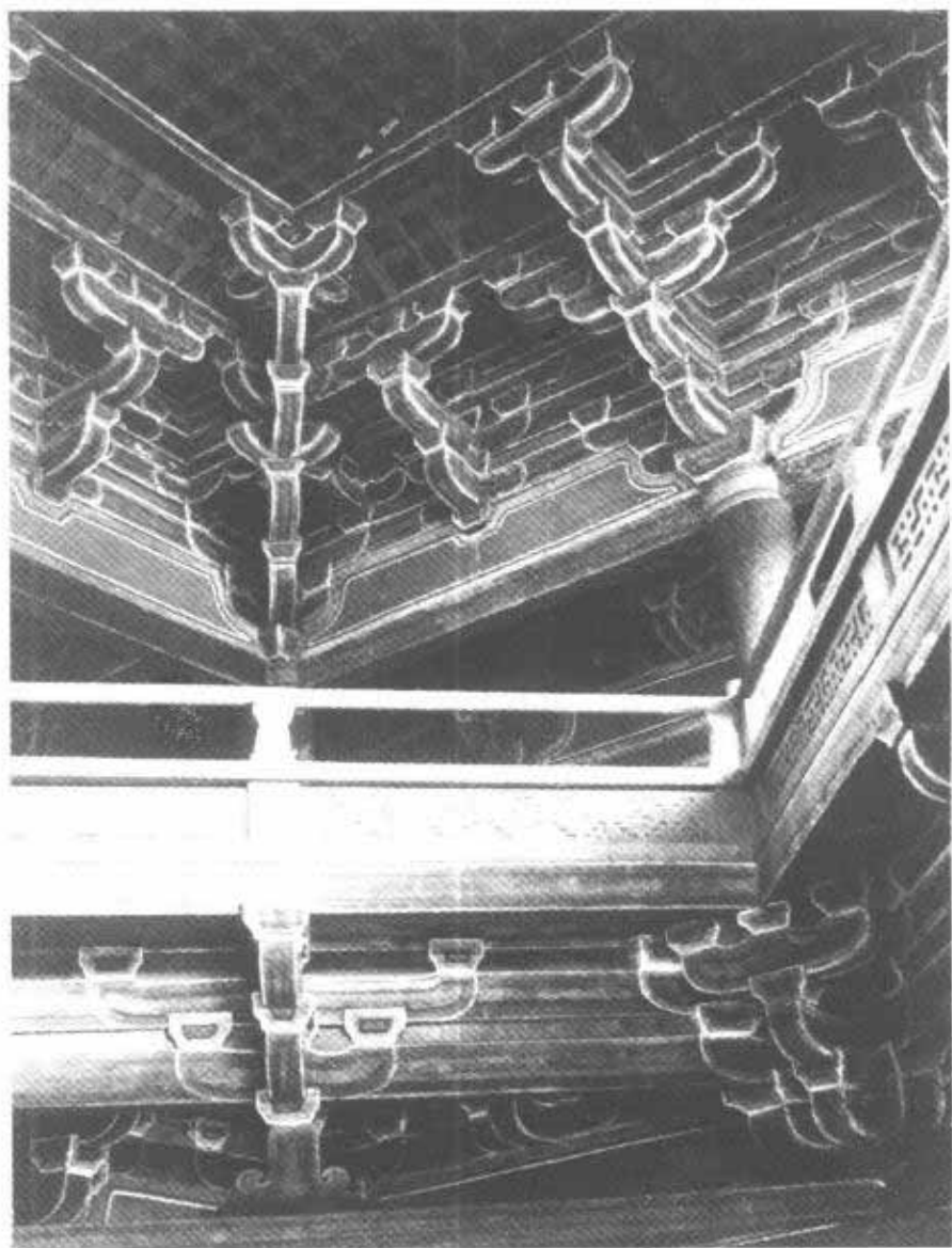
第41图 独乐寺观音阁内部斗拱
