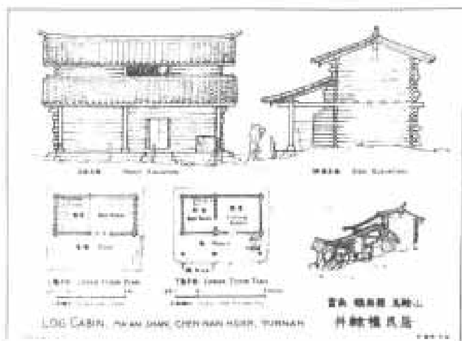
第 179 图 云南镇南井干式民居
